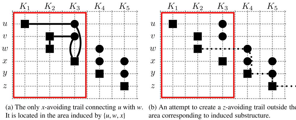
Fig. 5. Illustration of Lemma 2.17.
